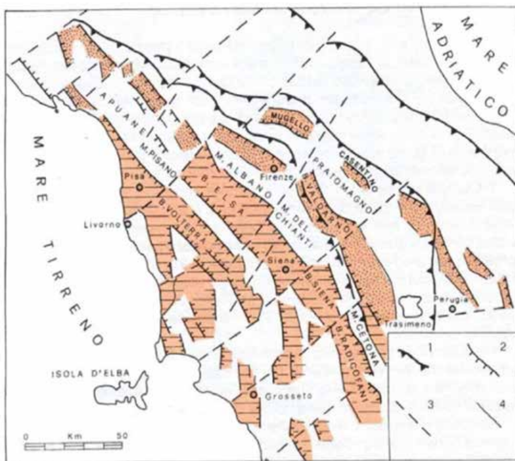
Figura 7: distribuzione dei principali bacini post-orogeni dell'Appennino settentrionale. In rigato sono indicati i bacini mio-pliocenici con depositi continentali e marini, in puntinato i bacini plio-pleistocenici con sedimenti continentali fluvio-lacustri. 1) principali fronti di accavallamento delle unità tettoniche appenniniche; 2) faglie principali al bordo dei bacini; 3) linee tettoniche trasversali; 4) faglie minori al bordo dei bacini. (da Martini & Sagri, 1993). Tratto da: Pandeli [5].
