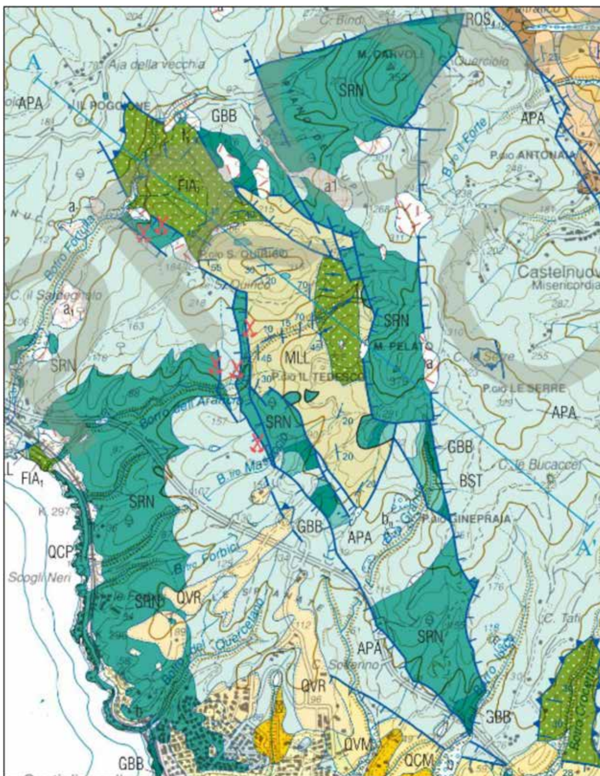
Figura 9: porzione del foglio 284 [6] di Rosignano Marittimo. Progetto CARG [7]. I colori e le sigle indicano varie litologie. La sigla SRN: serpentiniti (Giurassico medio), GBB: gabbri (Giurassico medio), BST: basalti (Giurassico superiore), FIA: membro del Fortulla (argilliti rosse e verdi in cui si intercalano siltiti e rocce calcaree, il membro è databile al Cenomaniano), MLL: formazione di Monte Morello (calcari grigi a grana fine, calcari marnosi, calcareniti, marne e argilliti, databili al Pleocene medio – Eocene medio), APA: argille a palombini (calcilutiti color grigio ferro in
