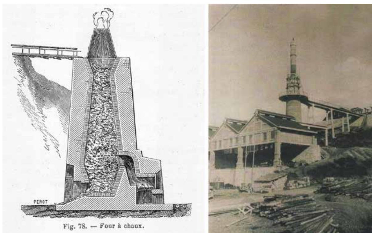
Figura 30: a sinistra schema di un forno a calce, a destra il forno di calcinazione della magnesite, posto a pochi metri dalla ferrovia.
