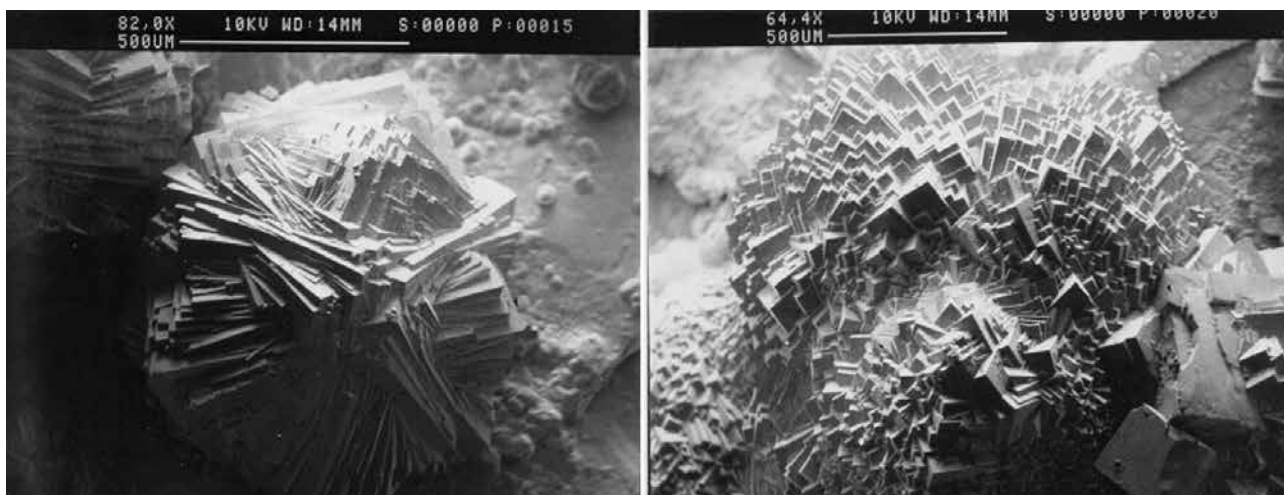
Figura 38a: aggregati polisintetici di individui cubici.
