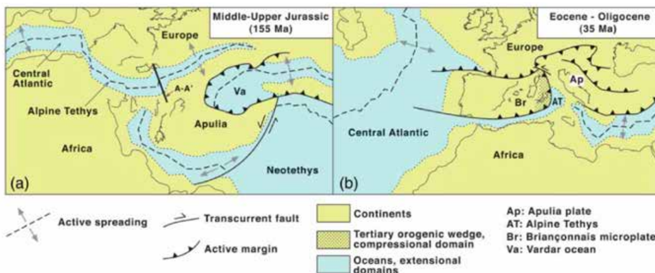
Figura 2: ricostruzione dell'area Mediterranea occidentale. L'oceano Tetide è indicato come AT (Alpine Tethys). Carmignani et al. 2013 [3].
